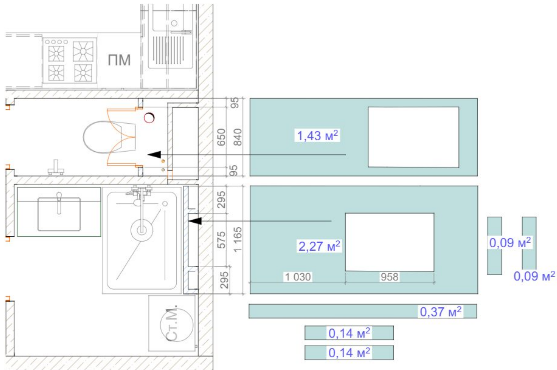
Схема розкладки ГКЛ.В
