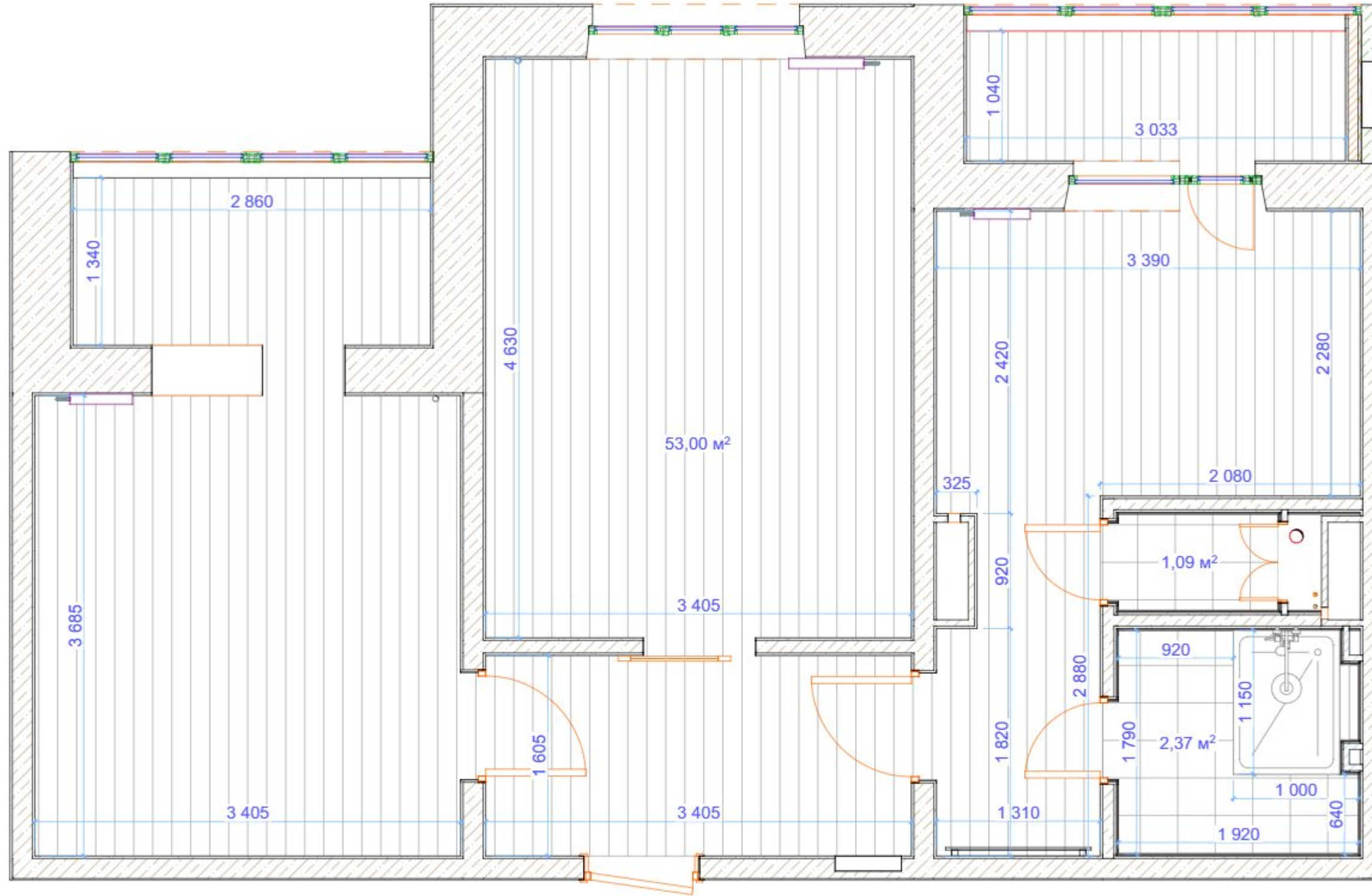
Схема підлогових покриттів
