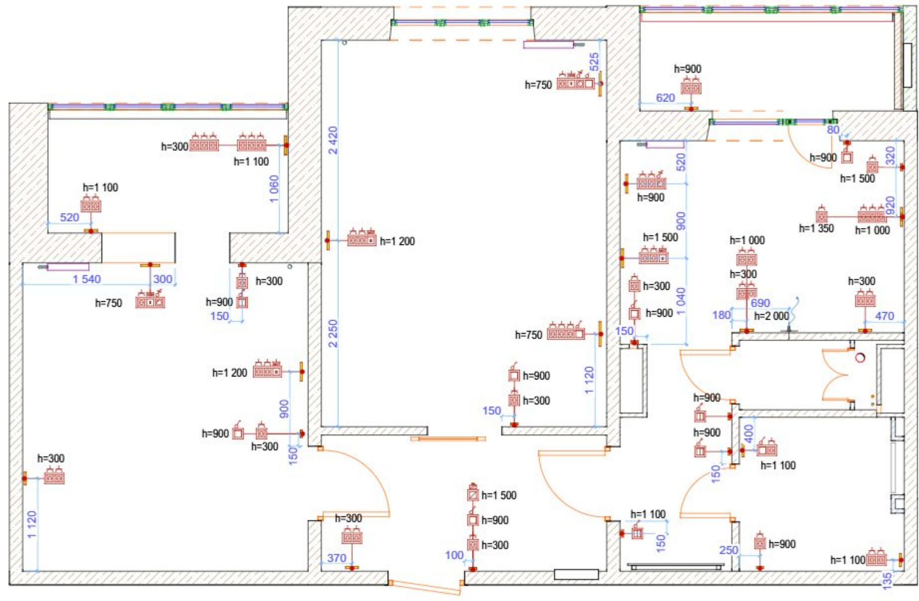
Схема розміщення електрофурнітури
