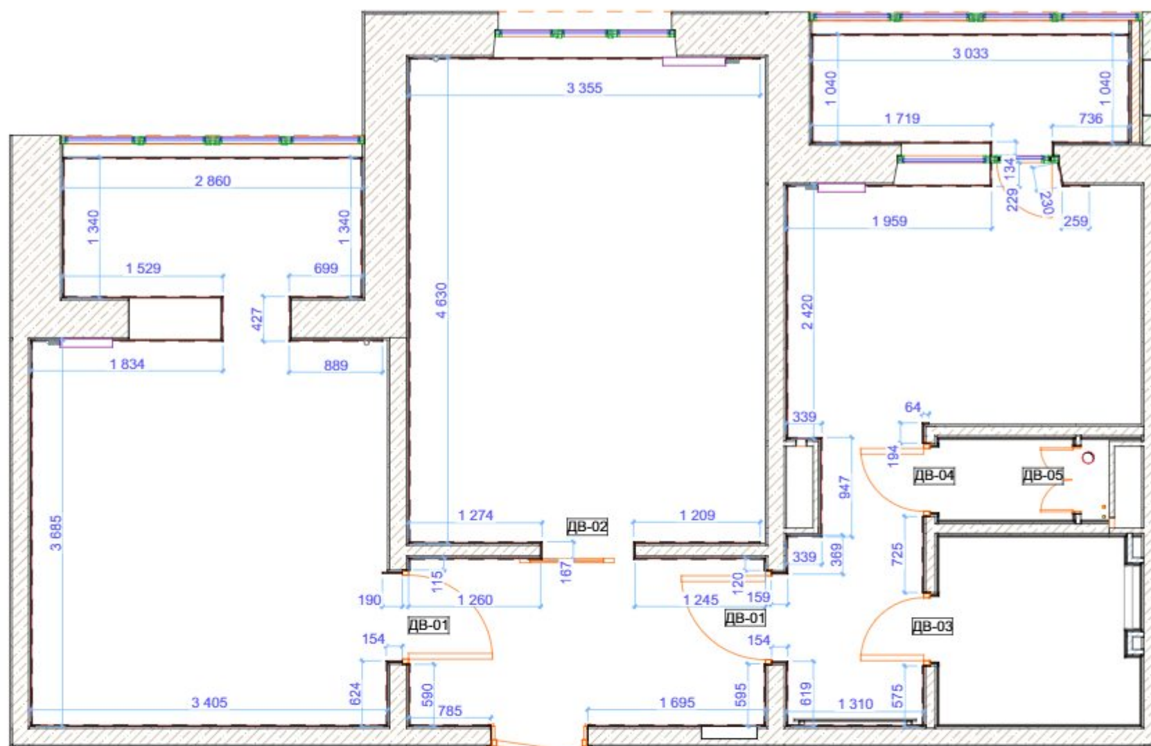
Схема розміщення плнтуса та специфікація дверей
